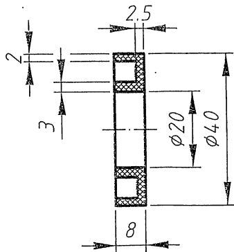
骨架式油封 20×40×8
