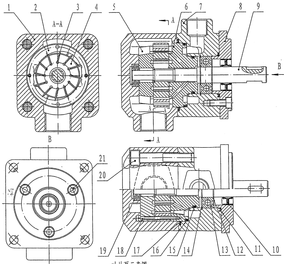
叶片泵示意图
