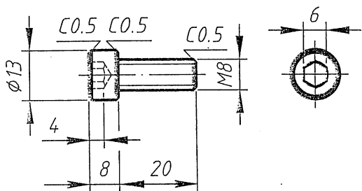
GB/T 70.1-2008 内六角圆柱头螺钉M8×20
