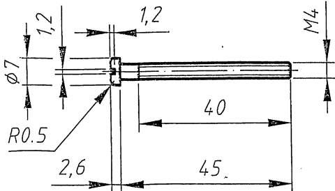
GB/T 65-2000 开槽圆柱头螺钉
