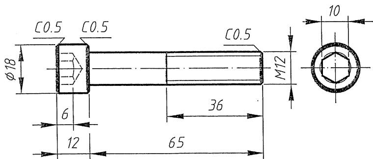
GB/T 70.1-2008 内六角圆柱头螺钉m12×65
