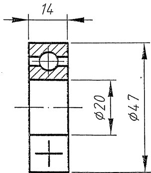
GB/T 276-1994 深沟球轴承
